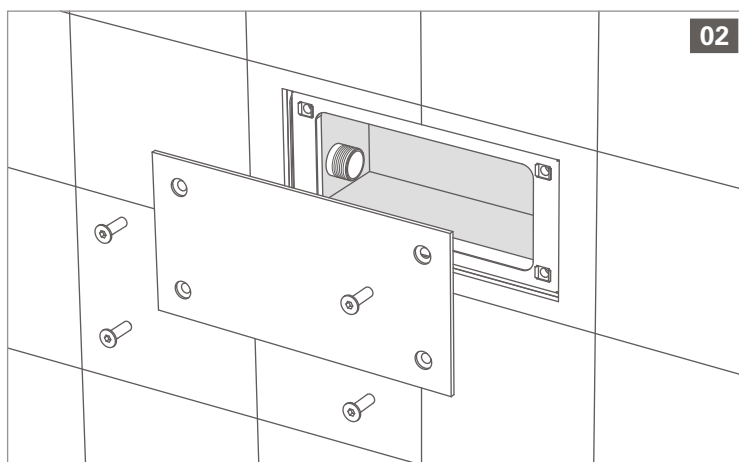
Montagem especial ligações de água do lado direito ou por baixo Special assembly water connections on the right side or below
