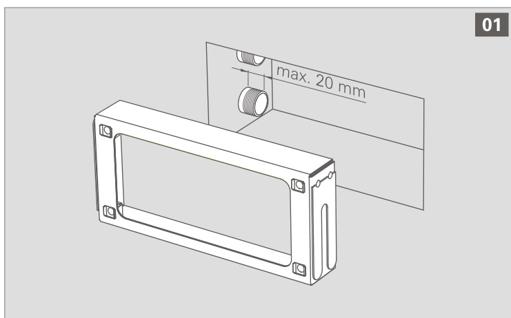
Montagem standard ligações de água do lado esquerdo Standard assembly water connections on the left side
