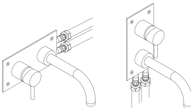
Montagem especial ligações de água do lado direito ou por baixo Special assembly water connections on the right side or below
