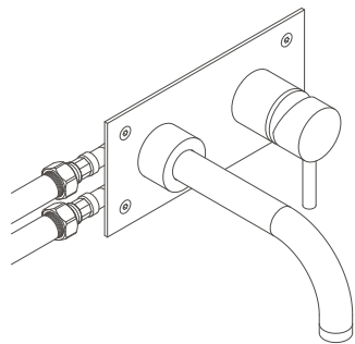
Montagem standard ligações de água do lado esquerdo Standard assembly water connections on the left side
