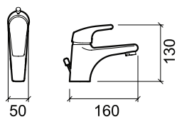
5364300 misturadora de lavatório sénior senior basin mixer mitigeur de lavabo senior
