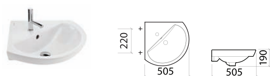
131700 lavatório canto compact corner basin lavabo d'algle
